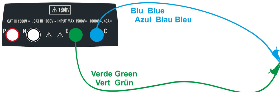
Fig. 5: Compensazione della resistenza dei cavi di misura
