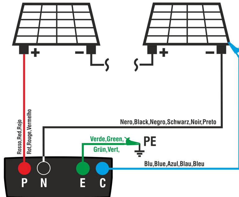
Fig. 10: Collegamento per test IVCK senza unità remota
